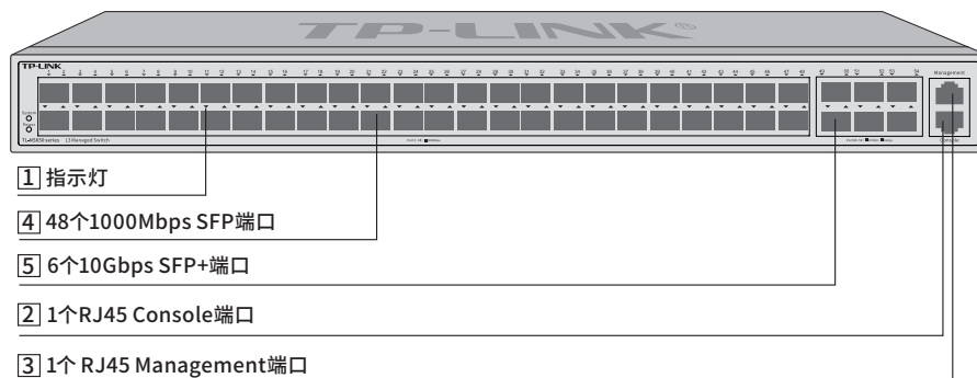
图1-4 TL-NS650-48F6T前面板示意图
