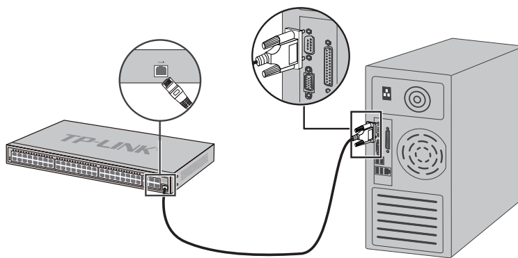
图3-3 RJ45 Console端口连接示意图
