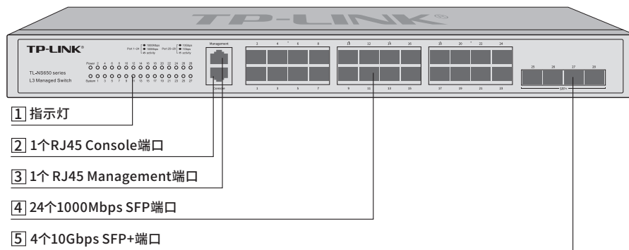
图1-3 TL-NS650-24F4T前面板示意图
