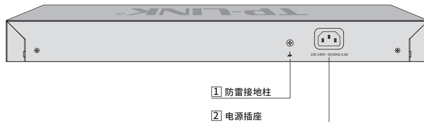
图1-6 后面板示意图
